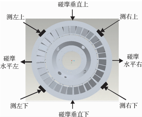
图 4 应变片位置及碰摩位置
