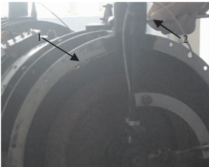
1 碰摩火花;2 拧碰摩螺钉产生碰摩
